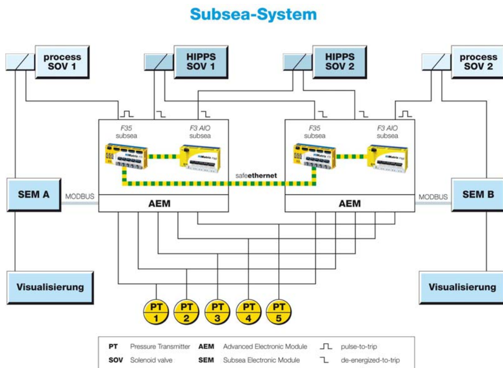
Bild 4 : Die Gesamtstruktur des Subsea-Systems wurde redundant ausgelegt.
