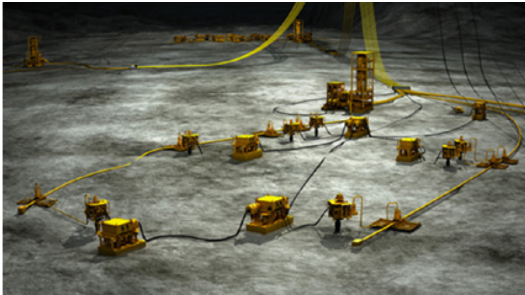
Bild 1: Quelle: FMC Technologies, Inc. Subsea Produkt- und Steuerleitungssystem
